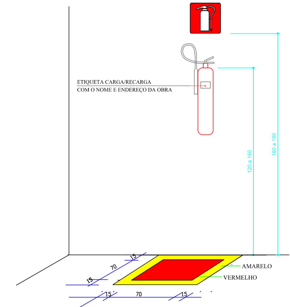
DET. SINALIZAÇÃO / EXTINTORES/INTERNO
